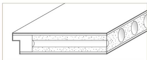
vratno krilo s sredico iz polne perforirane iverne plošče – RS
