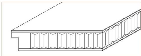
vratno krilo s sredico iz satja
